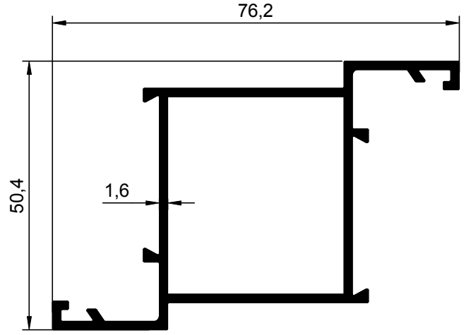
NO : 1183 AGIRLIK : 0.984 kg/m
