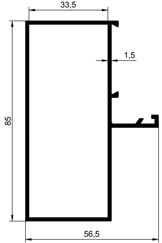
NO : 1407 AGIRLIK : 1.114 kg/m
