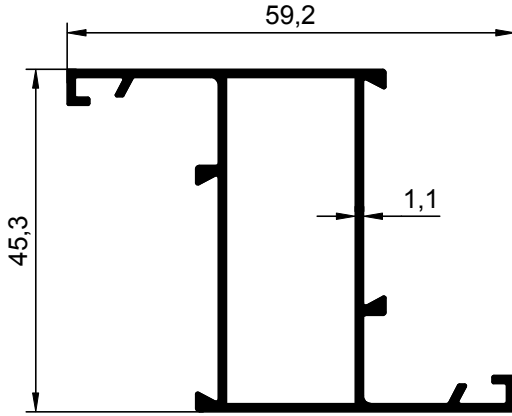
NO : 1346 AGIRLIK : 0.605 kg/m
