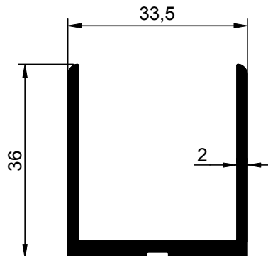
NO : 1396 AGIRLIK : 0.629 kg/m
