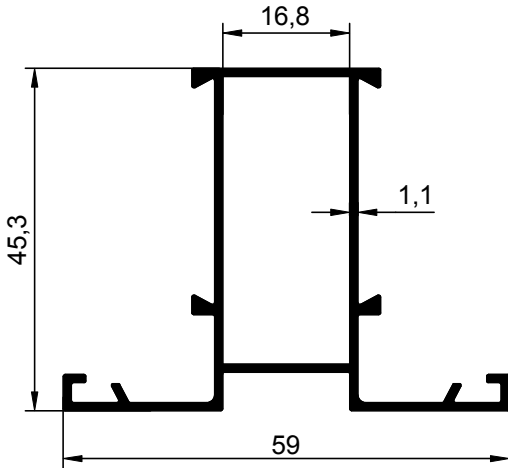
NO : 595 AGIRLIK : 0.602 kg/m
