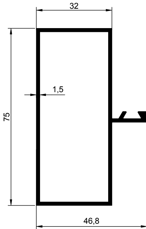
NO : 747 AGIRLIK : 0.941 kg/m
