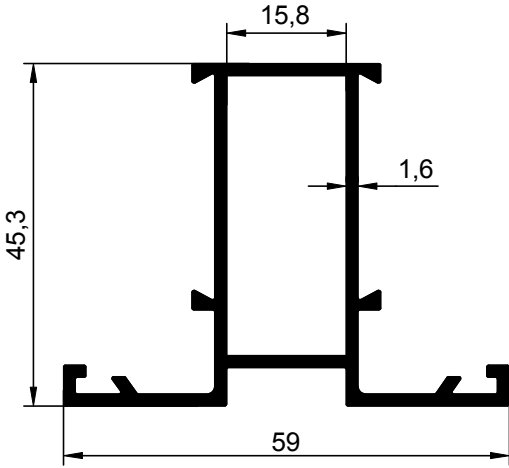
NO : 1203 AGIRLIK : 0.836 kg/m
