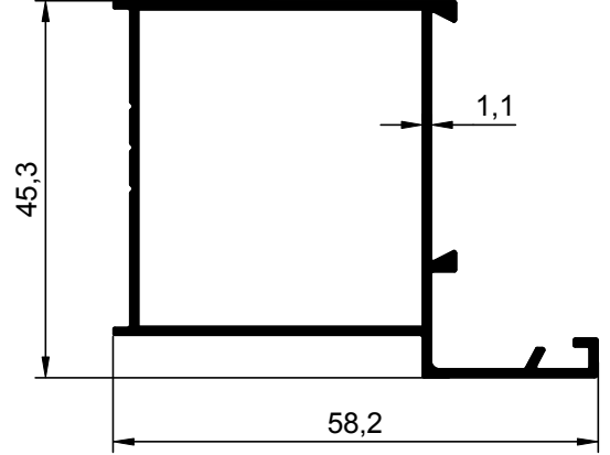
NO : 944 AGIRLIK : 0.583 kg/m
