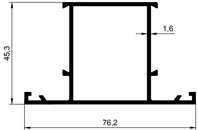
NO : 1578 AGIRLIK : 0.984 kg/m
