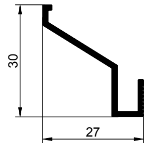
NO : 611 AGIRLIK : 0.225 kg/m
