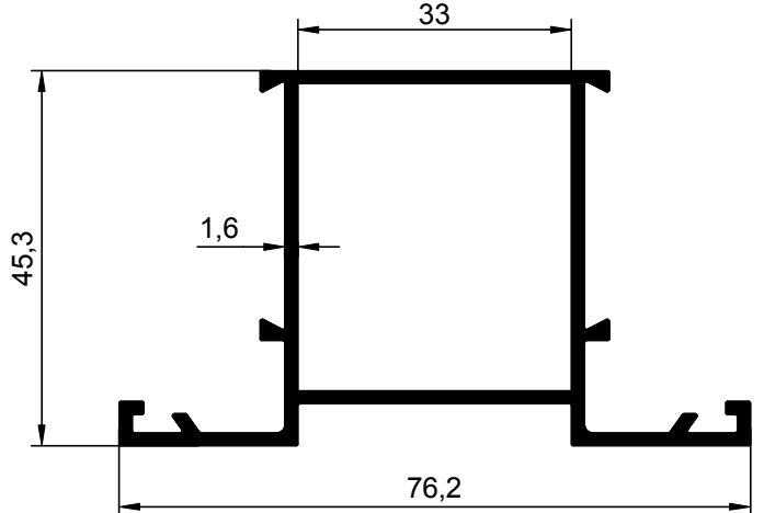
NO : 1181 AGIRLIK : 0.984 kg/m
