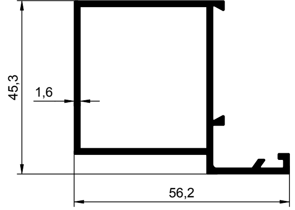
NO : 1182 AGIRLIK : 0.809 kg/m
