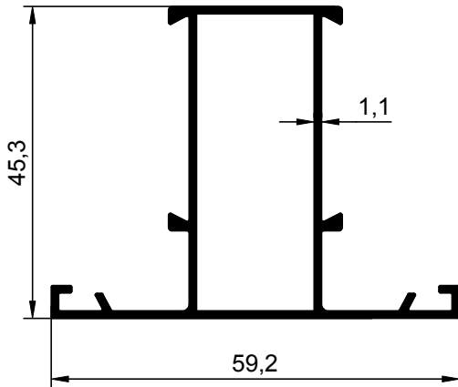
NO : 1345 AGIRLIK : 0.605 kg/m
