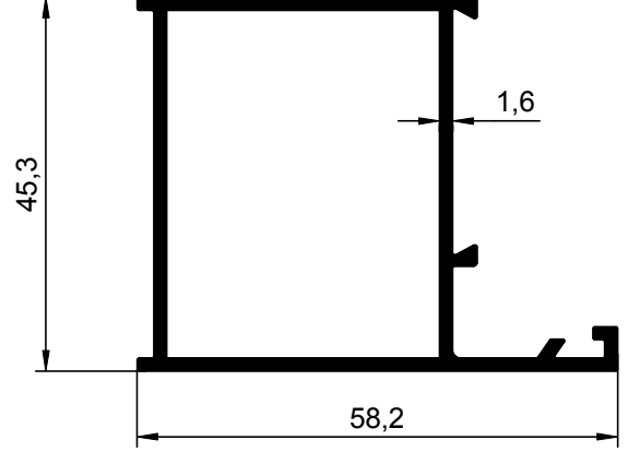
NO : 1577 AGIRLIK : 0.848 kg/m
