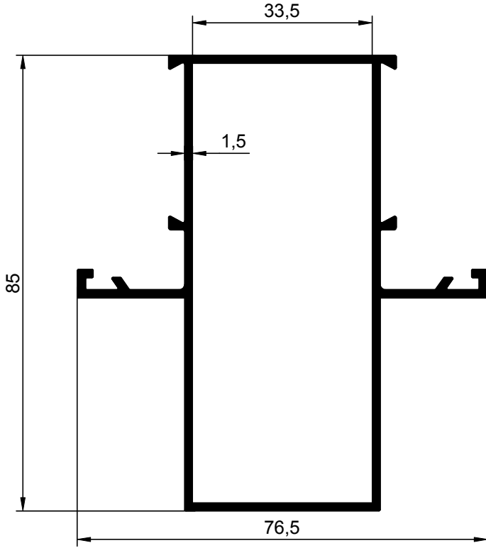
NO : 1122 AGIRLIK : .1.270 kg/m
