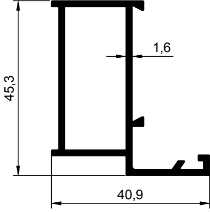
NO : 1205 AGIRLIK : 0.676 kg/m
