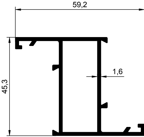
NO : 1139 AGIRLIK : 0.837 kg/m
