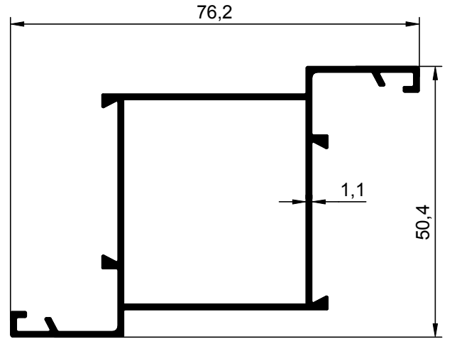
NO : 946 AGIRLIK : 0.705 kg/m
