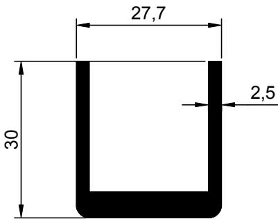
NO : 1133 AGIRLIK : 0.705 kg/m
